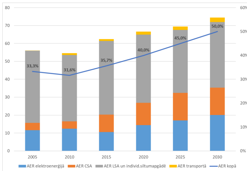
47.attēls. Mērķa scenārijā prognozētais AER īpatsvars enerģijas galapatēriņā (labā ass – %) un AER īpatsvara prognozes periodā līdz 2030.gadam (kreisā ass – PJ) 232
