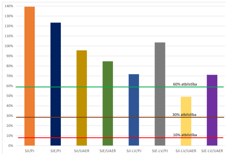
26.attēls. Latvijas elektroenerģijas starpsavienojumu līmenis 2018.gadā
